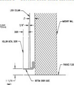
DETAIL D - BOTTOM DOOR GUIDE SECTION
