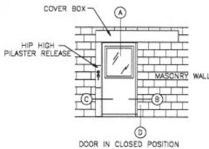
3165LX.bP-2 SLIDING DOOR SYSTEM
